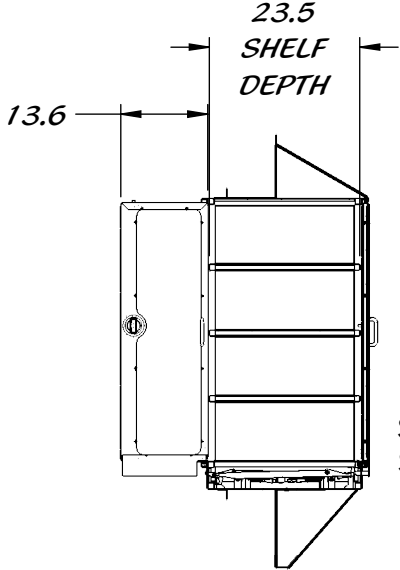
SECTION B-B SCALE 1 : 30
